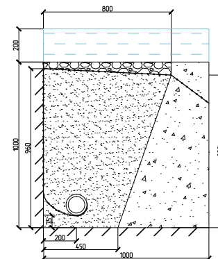
Рис. 2. Модифицированное решение пристенного дренажа с профилированной мембраной PLANTER Geo.
