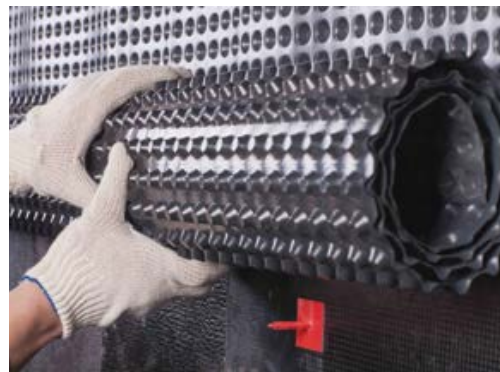
Защита гидроизоляции
